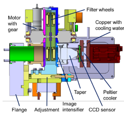
Fig. 6. Camera unit.
