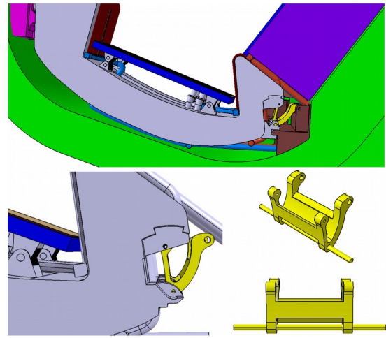
Fig. 11. Fixation option 2.
